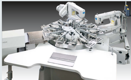
Dürkopp Adler 971-01 – Doppelkettenstich-Nähanlage zum Vornähen und Beschneiden von Manschetten durch Schablonensteuerung (~ 5.000 Manschetten in 480')
