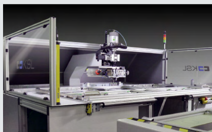
KSL 311 – CNC-Drehkopf-Nähanlage mit C-Bügel für Servo-motorisch gesteuertes, kontinuierliches oder intermittierendes Nähen frei programmierbarer Sicherheits-, Funktions- und dekorativer Nähte
