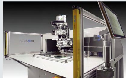
KSL 351 – CNC-Drehkopf-Portalnähanlage für Servo-motorisch gesteuertes, kontinuierliches oder intermittierendes Nähen frei programmierbarer Sicherheits-, Funktions- und dekorativer Nähte
