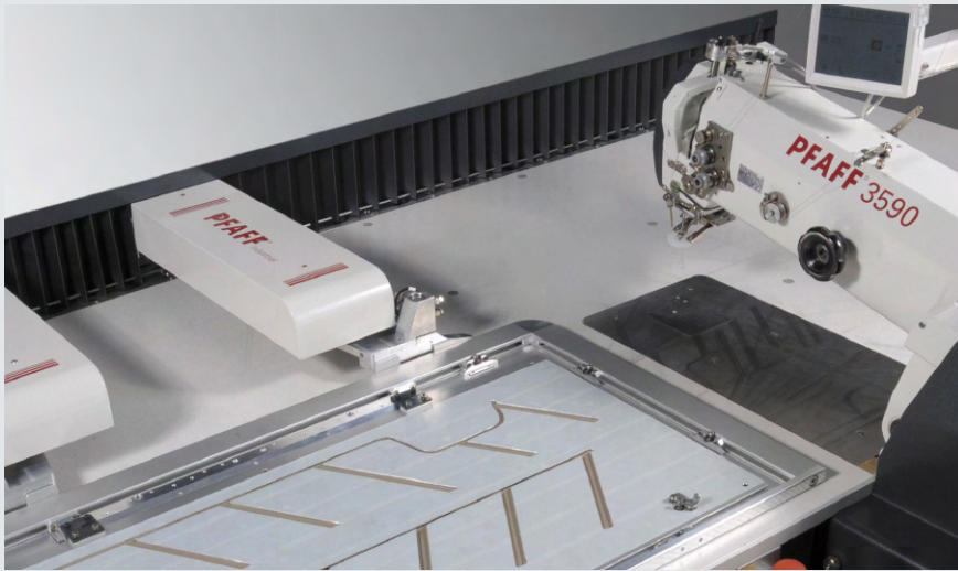
CNC-gesteuerte Nähanlage für dekorative Ziernähte CNC-controlled sewing unit for decorative seams
