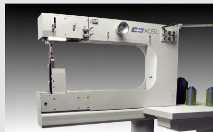
KSL 627 – Manuelle Kettenstich-Nähmaschine für das Nähen von Ziernähten bei der Innenausstattung von Automobilen wie Instrumententafeln, Türverkleidungen oder Armlehnen
